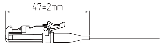
E2000 0.9>>Connector
